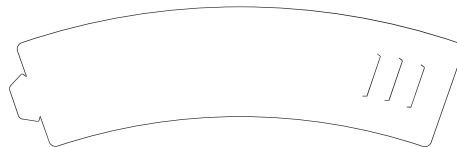
δαχτυλίδι κουμπωτό με 3 εγχοπές κατάλληλο για μεγέθη από 8 έως 16 oz
